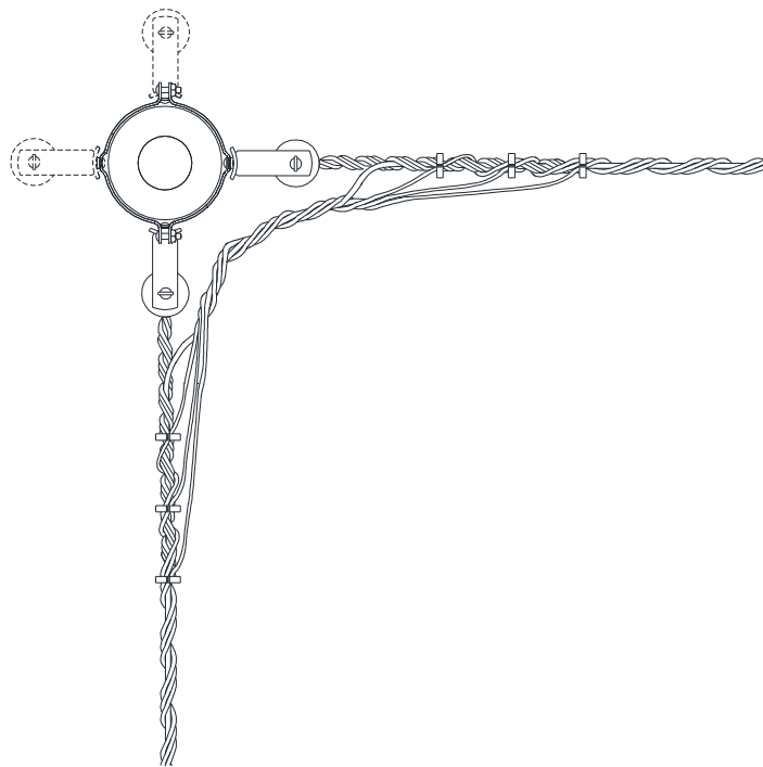
Figura 28 – Estrutura 90° - SI3 – SI3 (alternativa)
